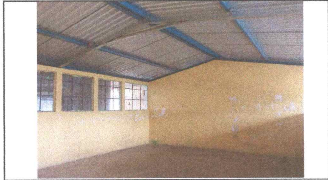
Foto 2: Se observa el deterioro de la estructura portante en el modulo 2
